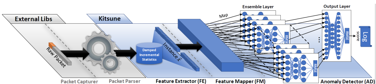
Figure 1 : Le système de détection d'intrusions Kitsune
